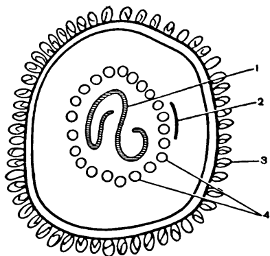
Рис. 5. Схема строения вирусной частицы (вириона):
