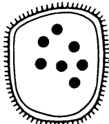
Рис. 3. Схематическое изображение относительных размеров и формы вирионов ДНК-содержащих и РНК-содержащих вирусов позвоночных: 1 — оспы; 2 — герпеса; 3 — аденовируса; 4 — паповавируса; 5 — парвовируса; 6 — ортомиксовируса; 7 — парамиксовируса; 8 — рабдовируса; 9 — тогавируса; 10 — буньявируса; 11 — аренавируса; 12 — ретровируса; 13 — коронавируса; 14 — пикорнавируса и 15 — реовируса.
