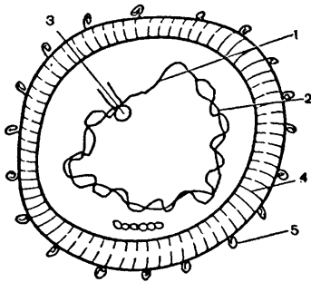
Рис. 11. Схема вириона вируса гепатита В;
